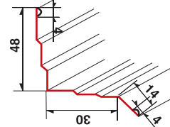
← 갈매기후레싱 90°
