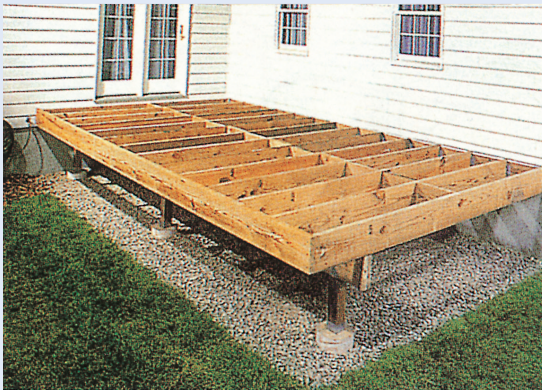
3 장선설치 - 장선고정 철물 사용 joist hanger
