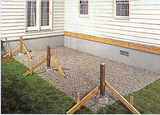
1 틀잡기 - 주춧돌/포스트베이스용 철물이용 정확한 수평·수직 시공
